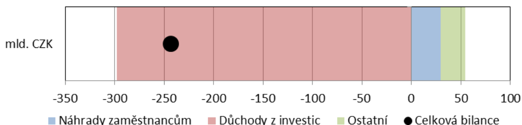
Graf 8 Bilance primárních důchodů podle typu důchodu v roce 2015. Záporné číslo značí odtok do zahraničí, výsledná čísla jsou dílčí bilancí (net). Zdroj: Databáze ARAD, ČNB
